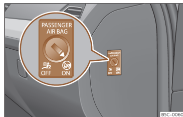
Fig. 26 Interruttore a chiave per l'attivazione e la disattivazione dell'airbag del passeggero.
