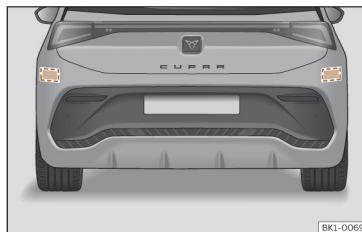
Fig. 105 Veduta posteriore del veicolo: zone dei sensori radar.
