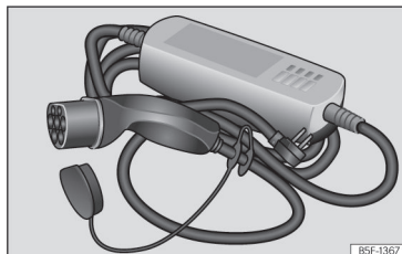
Fig. 60 Cavo di ricarica per prese di corrente.
