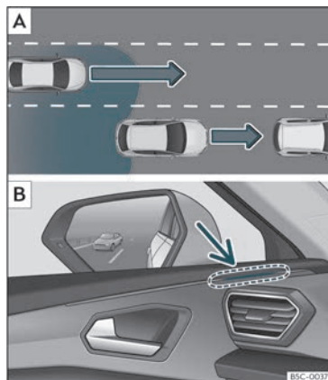
Fig. 170 Rappresentazione schematica: A ) Situazione in un sorpasso con traffico sulla parte posteriore. B ) Indicazione dell'assistente al cambio corsia sulla spia di controllo sinistra.
