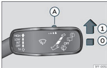
Fig. 95 Leva del tergicristalli: Regolazione del sensore pioggia A .
