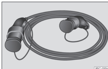
Fig. 195 Cavo di ricarica per stazioni di ricarica con corrente alternata (CA).
