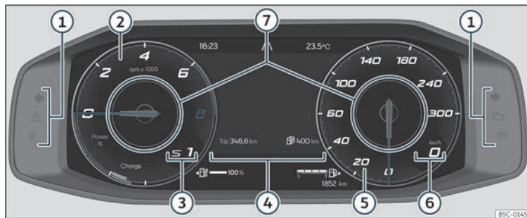
Fig. 52 Digital Cockpit nella plancia (visualizzazione classica).
