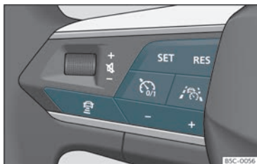
Fig. 167 Lato sinistro del volante multifunzione: tasti per la gestione del Travel Assist.
