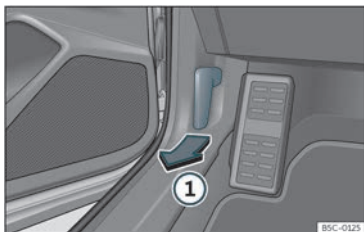
Fig. 201 Leva di sblocco nel vano piedi del lato conducente.
