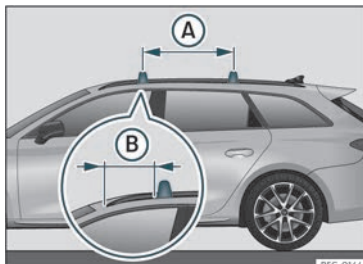
Fig. 125 Punti di fissaggio delle barre longitudinali per il portapacchi sul tetto.
