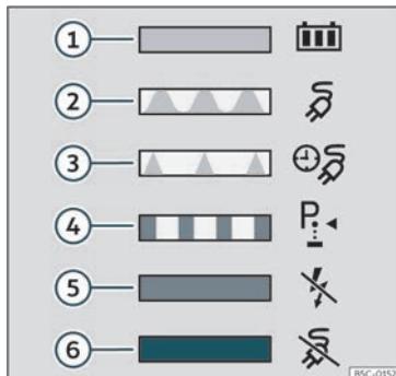
Fig. 193 All'interno del coperchio della presa di carica della batteria: adesivo con informazioni sull'indicatore del processo di ricarica.
