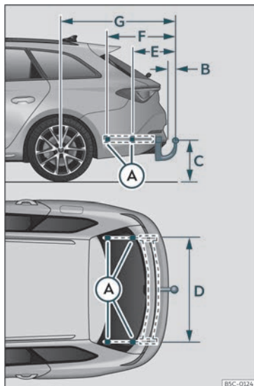
Fig. 188 Quote e punti di fissaggio per il montaggio successivo di un dispositivo di traino.
