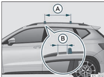
Fig. 123 Punti di fissaggio delle barre longitudinali per il portapacchi sul tetto.
