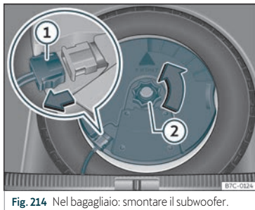
Fig. 214 Nel bagagliaio: smontare il subwoofer.
