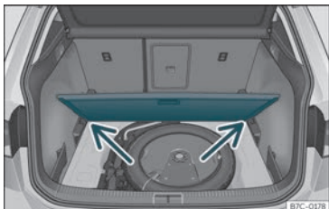
Fig. 115 Piano variabile del bagagliaio: posizione inclinata.
