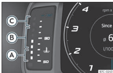
Fig. 61 Indicatore della temperatura del liquido di raffreddamento del motore.
